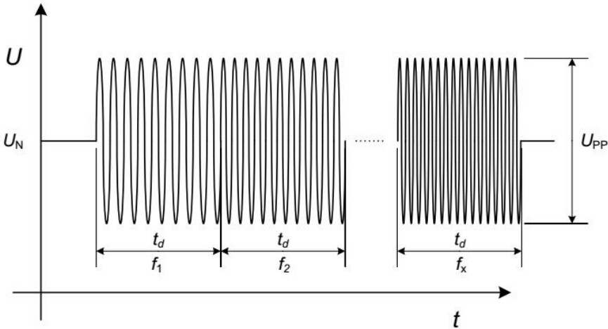
图B.2 试验脉冲B（低频正弦波骚扰）
