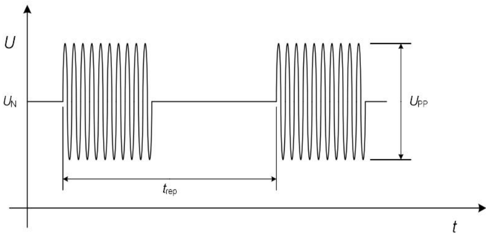
图B.1 试验脉冲A（正弦波脉冲），例如在HV+线上 表 B.2 试验脉冲 A（脉冲正弦波骚扰）的参数
